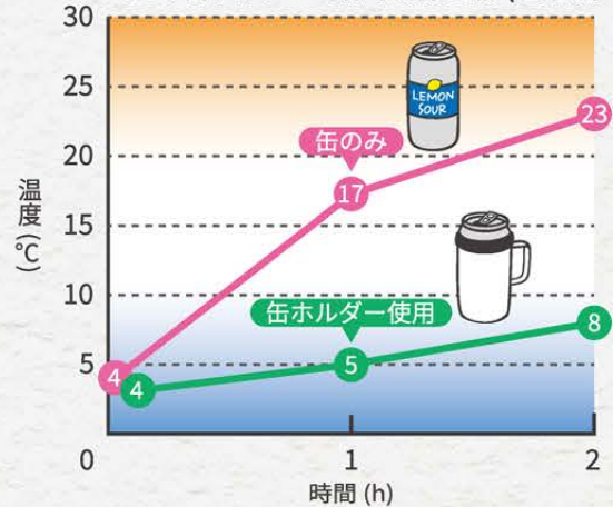
500ml 缶ホルダーの保冷効果比較 (当社調べ)
